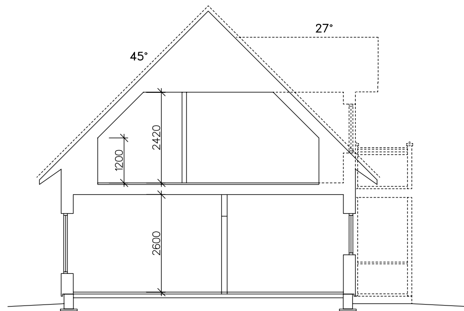
SCHNITT
