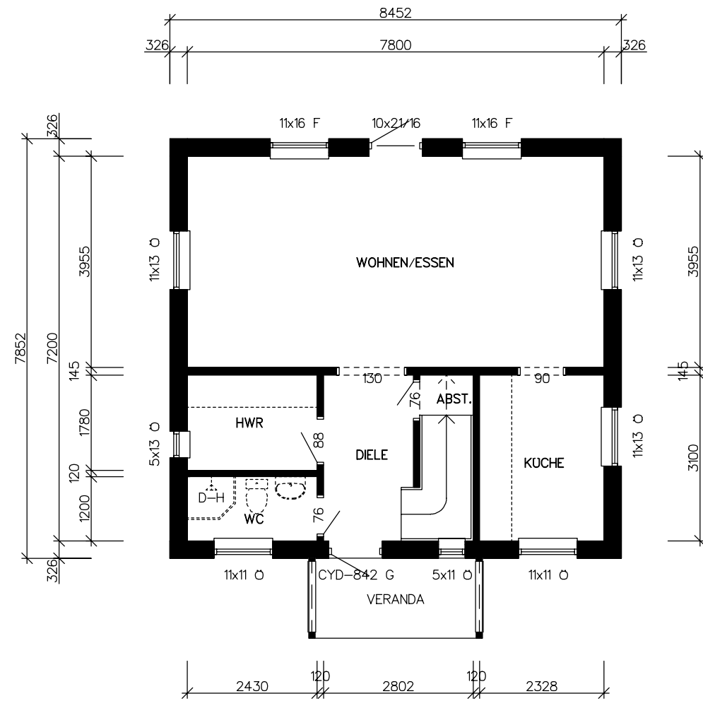
ERDGESCHOSS
