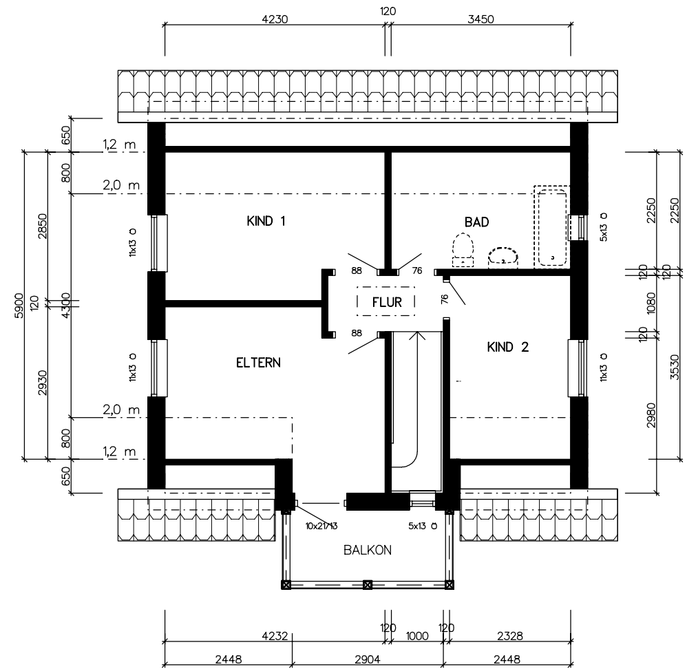
DACHGESCHOSS
